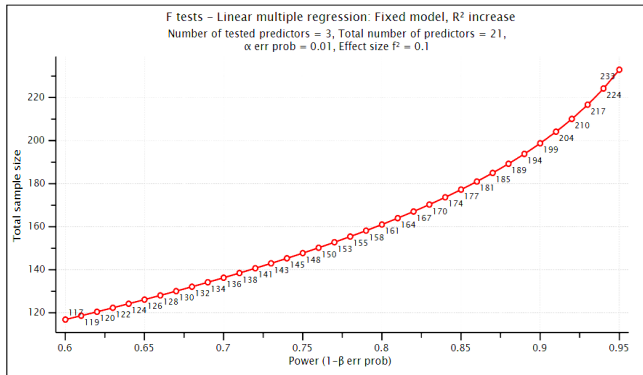
شکل ۱. نمودار بر آورد حجم نمونه
