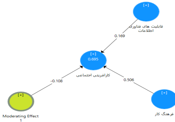
شکل ۲. مدل تحلیل مسیر در حالت ضرایب استاندارد
